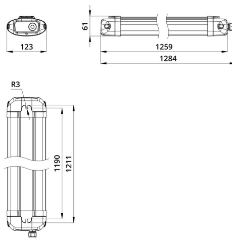
Габаритный чертеж
