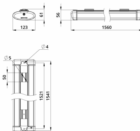
Габаритный чертеж
