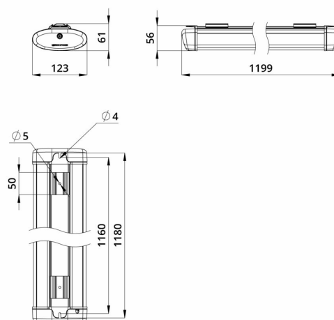
Габаритный чертеж
