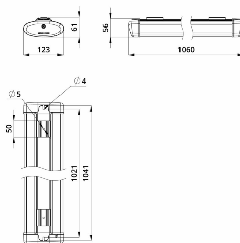
Габаритный чертеж
