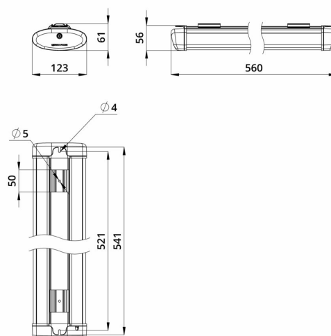
Габаритный чертеж
