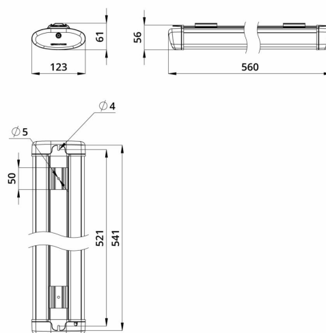
Габаритный чертеж
