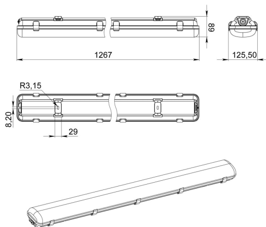
Габаритный чертеж
