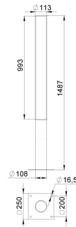
Габаритный чертеж
