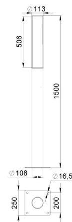
Габаритный чертеж
