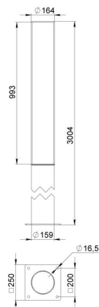
Габаритный чертеж
