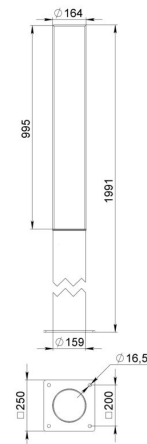
Габаритный чертеж
