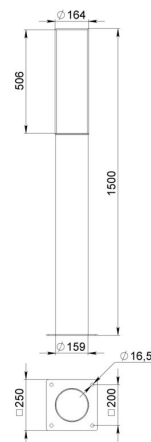
Габаритный чертеж
