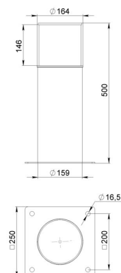
Габаритный чертеж
