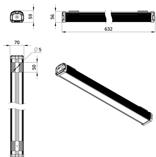
Габаритный чертеж
