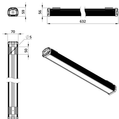
Габаритный чертеж
