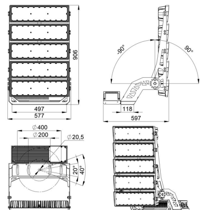
Габаритный чертеж
