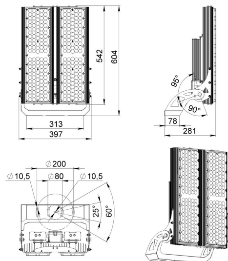
Габаритный чертеж
