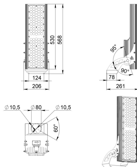
Габаритный чертеж
