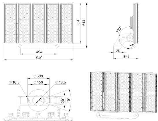
Габаритный чертёж
