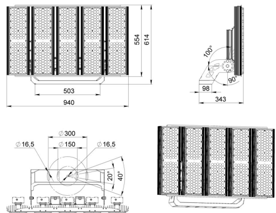
Габаритный чертеж
