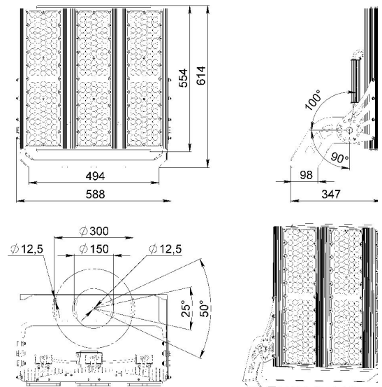
Габаритный чертёж
