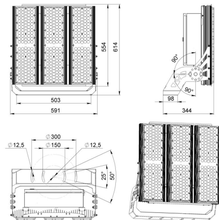
Габаритный чертеж
