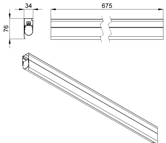
Габаритный чертеж
