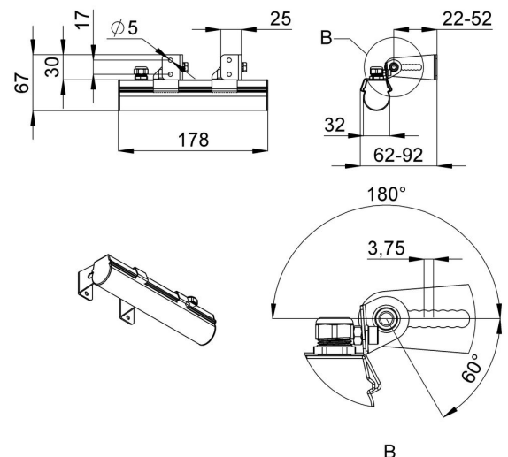
Габаритный чертеж
