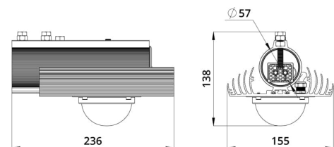
Габаритный чертеж
