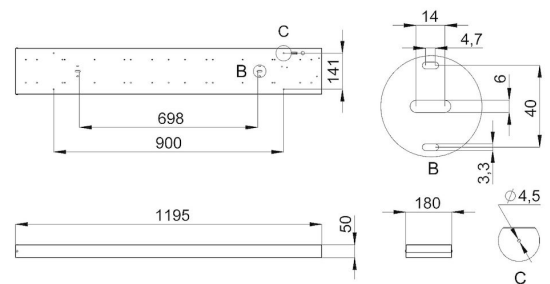
Монтаж светильника
