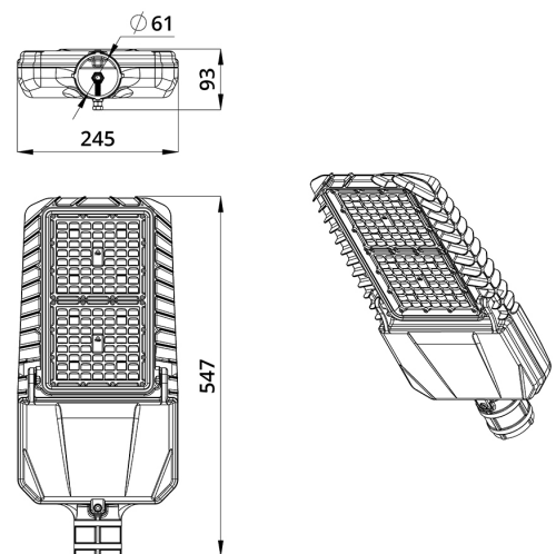
Габаритный чертеж
