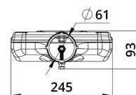
Габаритный чертеж
