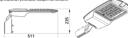
Угол регулировки поворотной консоли \pm 15^\circ с шагом 5^\circ .
