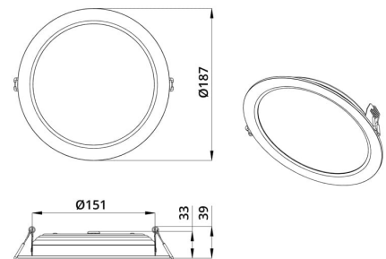
Монтаж светильника
