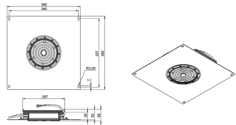
Монтаж светильника
