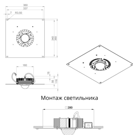
Габаритный чертёж
