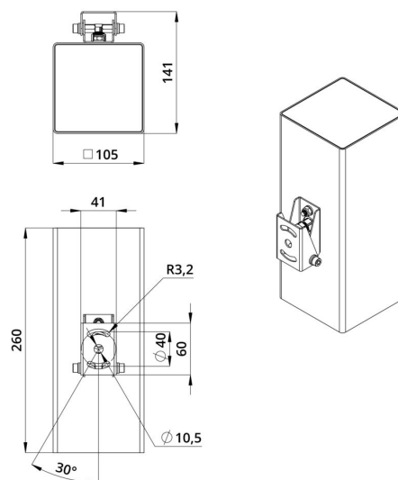
Габаритный чертеж
