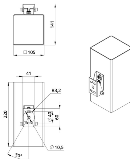
Габаритный чертеж
