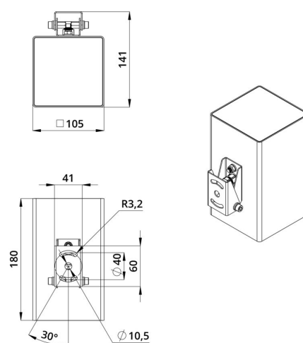
Габаритный чертеж
