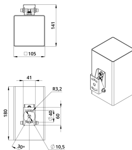
Габаритный чертеж
