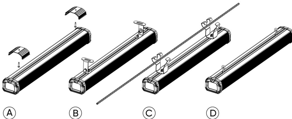
А – J-Hook, В – кронштейны, С – крепления на трос, D – винт-петли.
